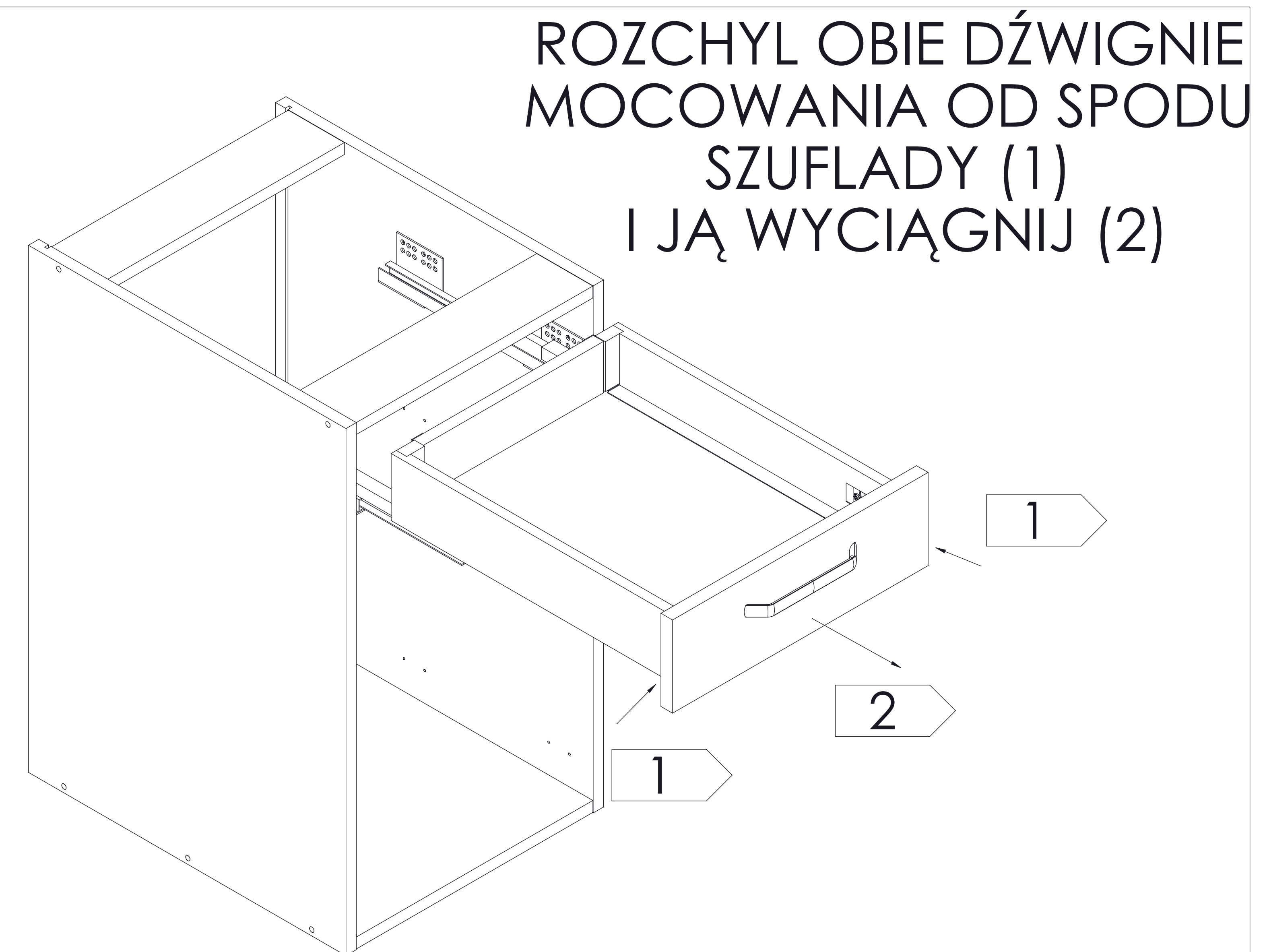
DEMONTAŻ SZUFLADY
