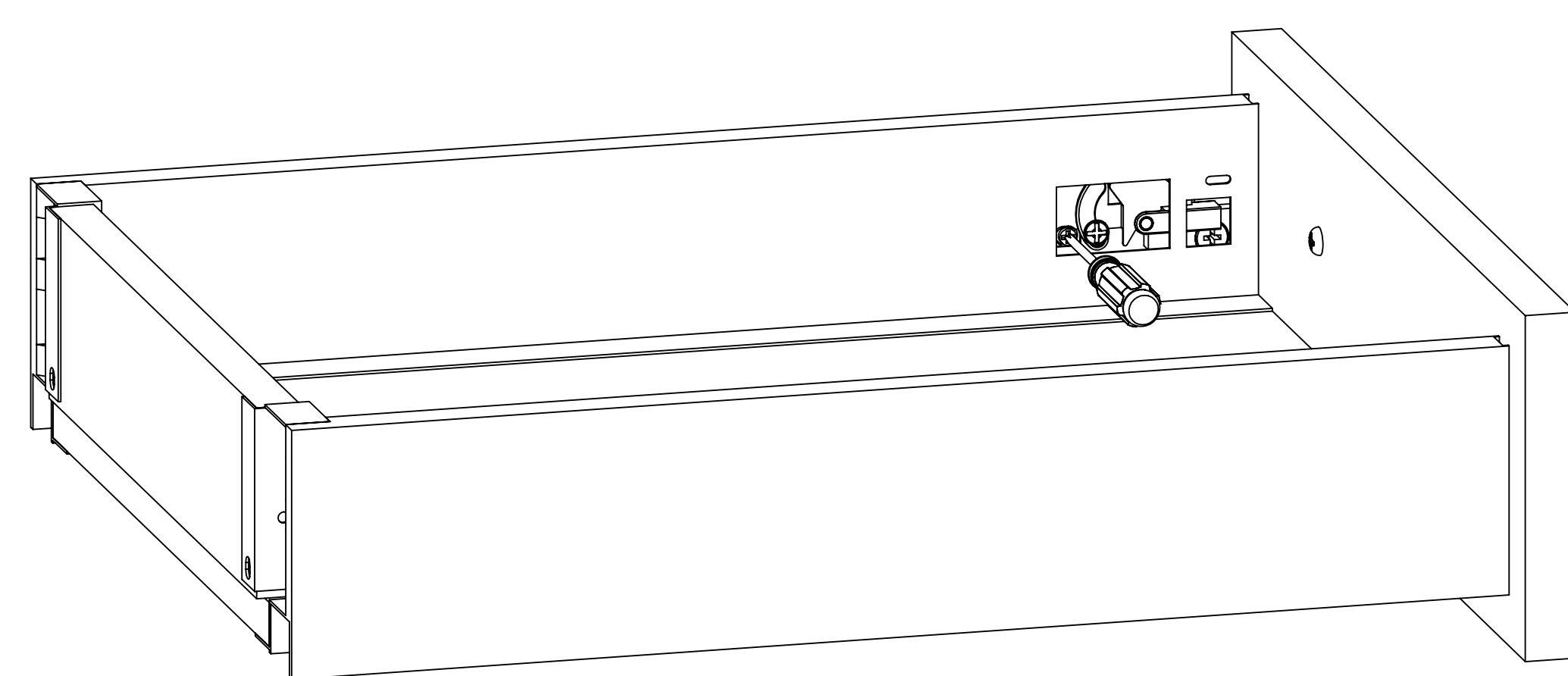
REGULACJA SZUFLADY
